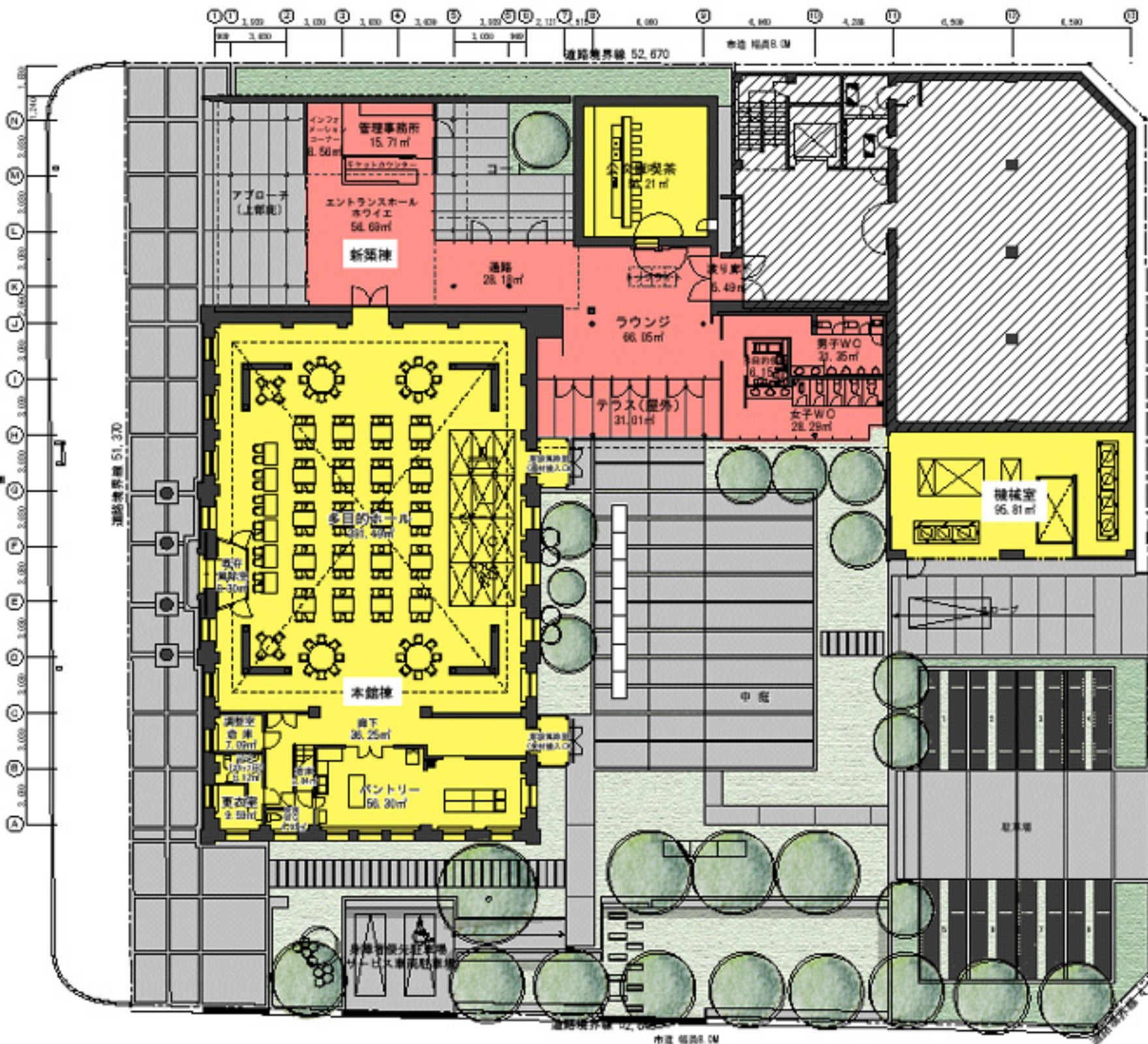
1階平面図 S=1/200
